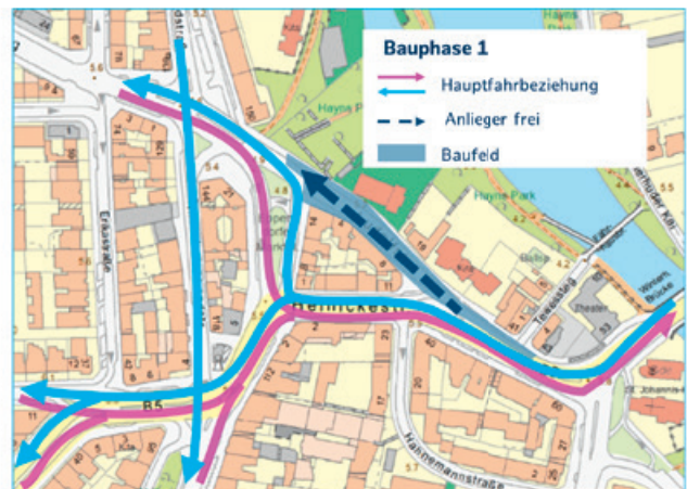
Abb. 2 Verkehrsführung in Bauphase 1 im Bereich Ludolfstraße Quelle: LGV/FHH-Atlas
