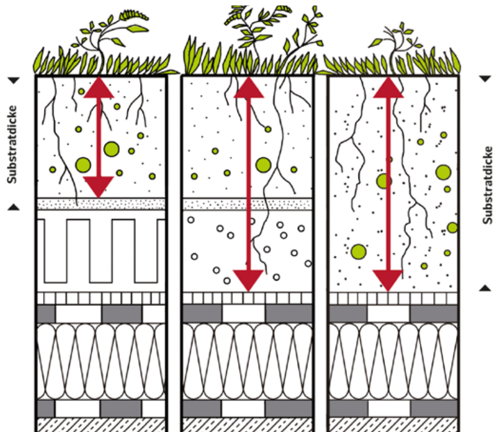
Schematischer Aufbau einer Dachbegrünung
