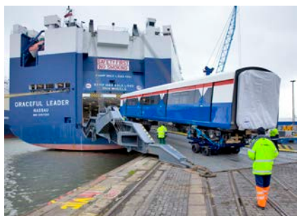
Verladung eines Metro-Waggons auf das RORO-Schiff NYK Graceful Leader am BLG-Autoterminal Bremerhaven
