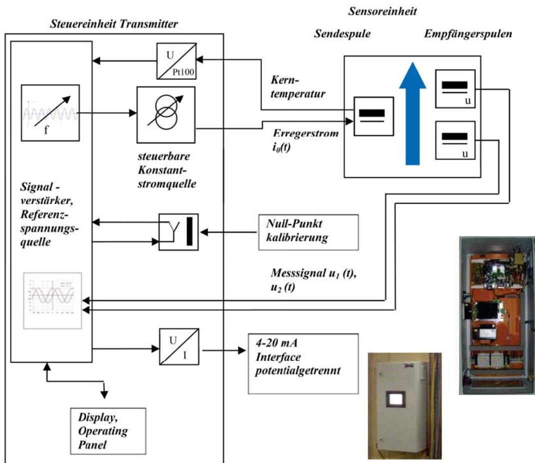
Abb.4: EMDps Steuereinheit [5]
