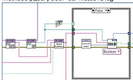
Methode „Query Bool“ der Klasse IOTag
