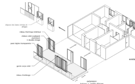
Prinzip der Erweiterung, Zeichnung: Lacaton&Vassal, Druot, Hutin, Bordeaux 2016.
