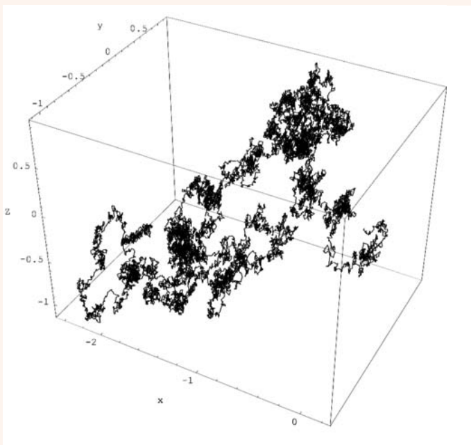
Einer von unendlich vielen gleich wahrscheinlichen Pfaden, die im Feynman'schen Pfadintegral eingesetzt werden
