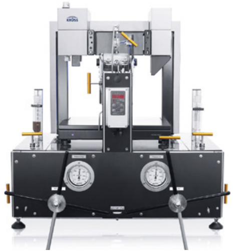
Kontaktwinkelmessgerät DSA100HP zur Messung auf Oberflächen unter extremen Drücken und Temperaturen
