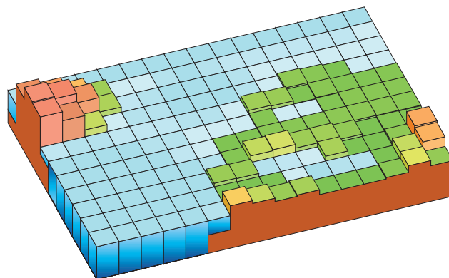
Räumliche Auflösung: Ausschnitt des Rechengitters für Europa, Gitterabstand ca. 500 km
