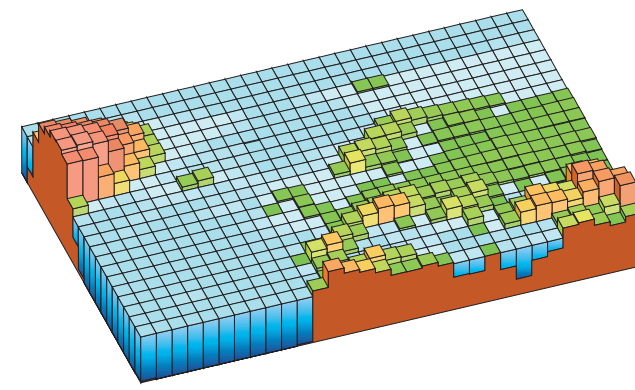
Gitterabstand ca. 250 km
