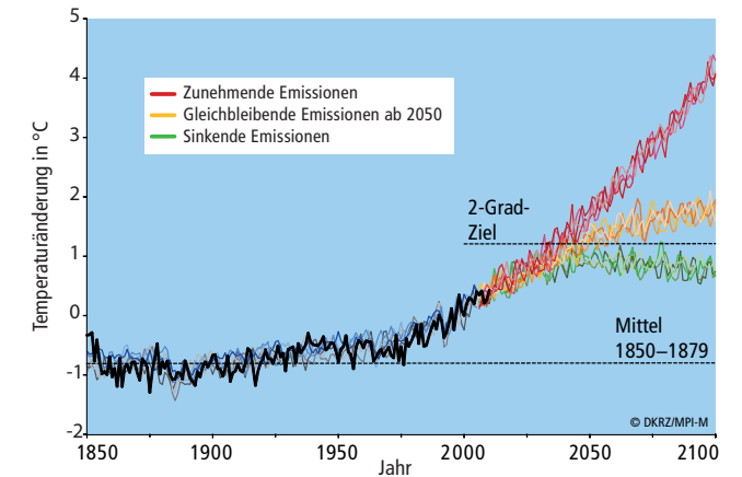
Ensembles: Mehrere Berechnungen zur Änderung der globalen mittleren Jahrestemperatur gegenüber 1986 bis 2005 mit einem Modell des Max-Planck-Instituts für Meteorologie in Hamburg
