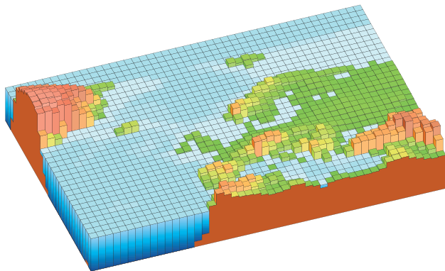
Gitterabstand ca. 180 km
