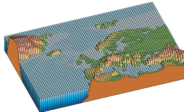
Gitterabstand ca. 110 km
