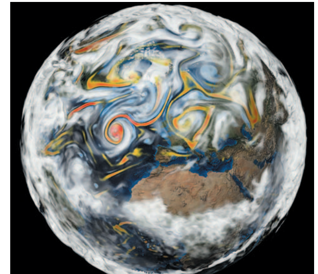
Dieses hochauflösende Klimamodell zeigt die Bewölkung und die Wirbelstärke.
