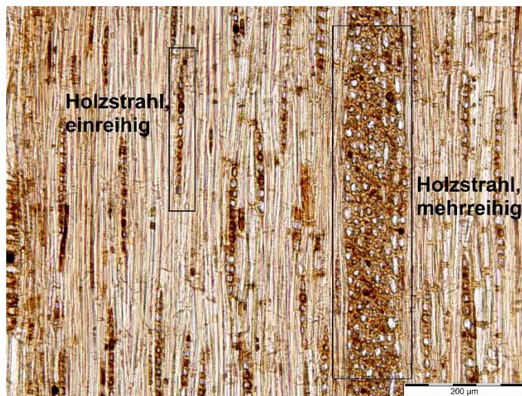
Abbildung 4-3: Eiche, Tangentialschnitt
