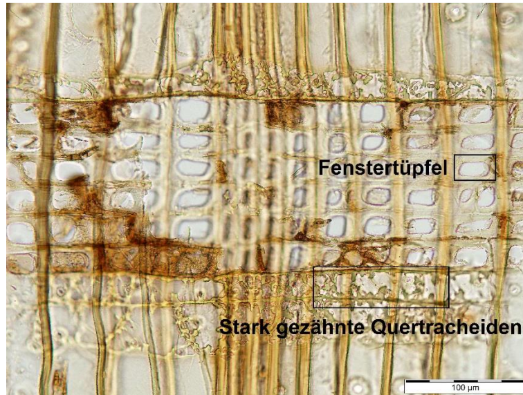
Abbildung 4-5: Kiefer, Radialschnitt
