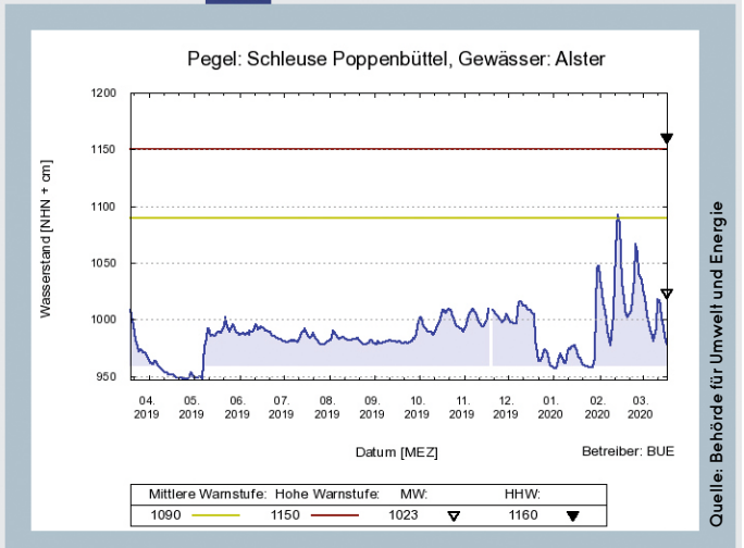
WASSERSTANDSGANGLINIEN SCHLEUSE POPPENBÜTTEL - ALSTER
