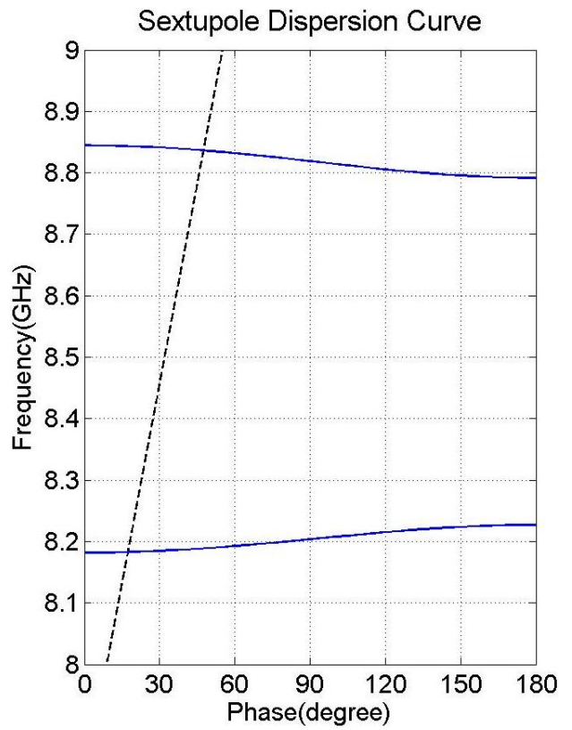
(d) Sextupole
