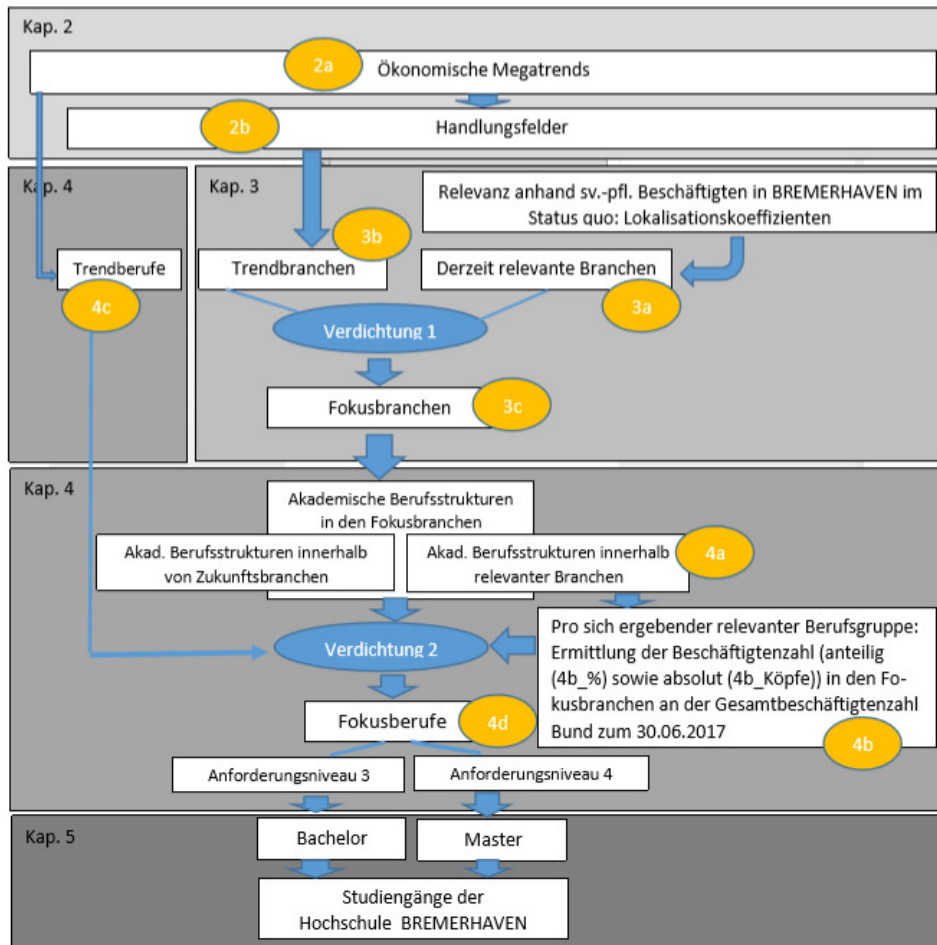
Abbildung 1: Methodische Vorgehensweise
