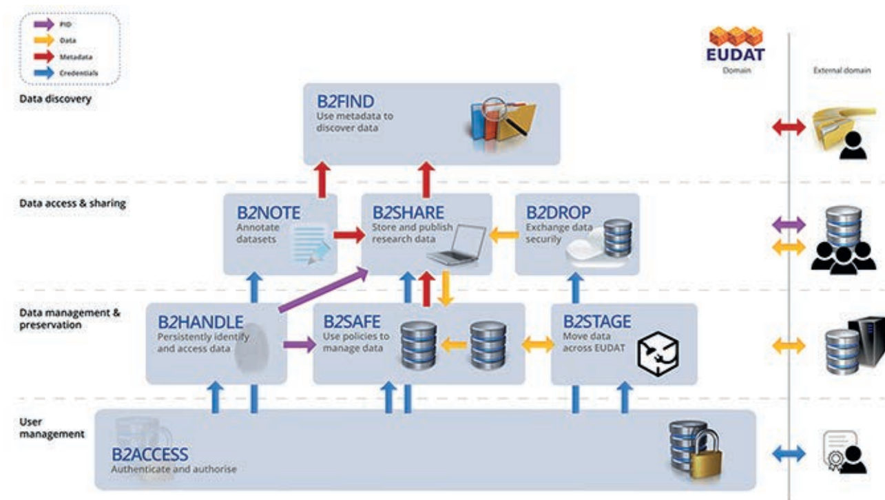
Abb. 2: Die Elemente der EUDAT-B2-Suite vereinfachen das Management wissenschaftlicher Daten. Das DKRZ beteiligte sich insbesondere an der Entwicklung der Dienste B2FIND und B2HANDLE.
