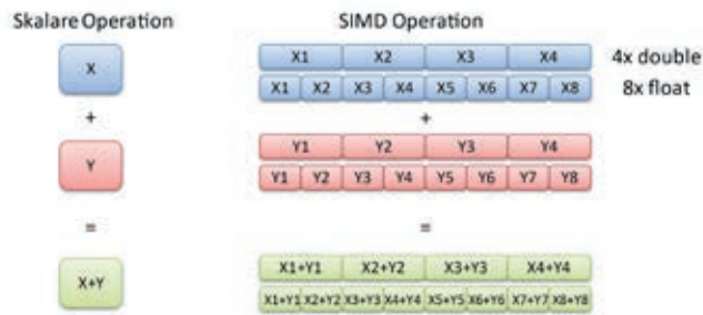
Abb. 2: Durch die Reduktion von doppelter (double) auf einfache Genauigkeit (float) kann die Anzahl paralleler Operationen verdoppelt werden.
