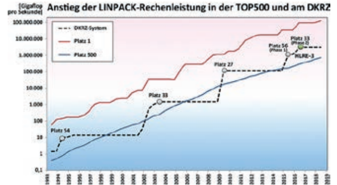
Abb. 4: Seit 1993 ist die Rechenleistung in der TOP500 und am DKRZ etwa um das 1.000.000-fache gestiegen. Das Hochleistungsrechnersystem für die Erdsystemforschung „Mistral“ stieg auf der Juni 2016-Liste der TOP500 auf Platz 33 ein.
