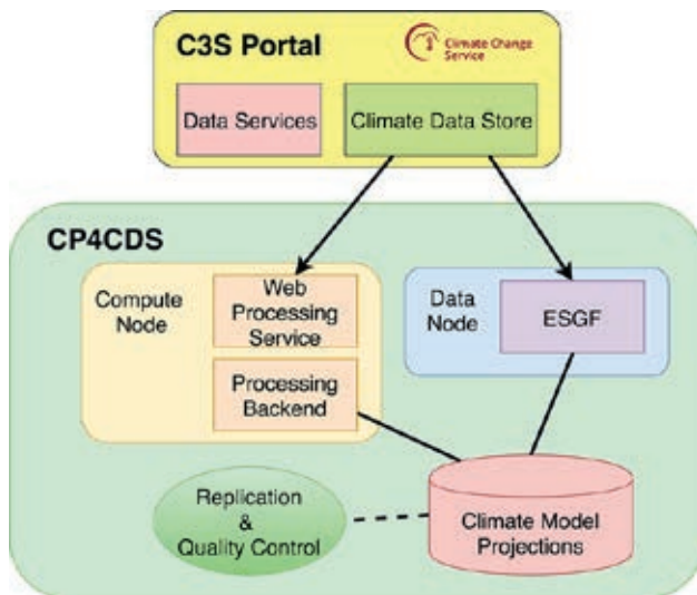
Abb. 1: Klimaprojektionen für den Copernicus-Klimadatenspeicher
