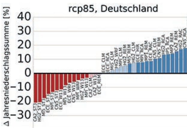
Abb. 2: Änderung (2070/2099 gegenüber 1971/2000) der Jahresniederschlagssumme in Deutschland (RCP8.5) bei verschiedenen Modellkonstellationen.
