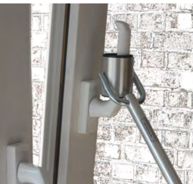
mobiler Fensteröffner
