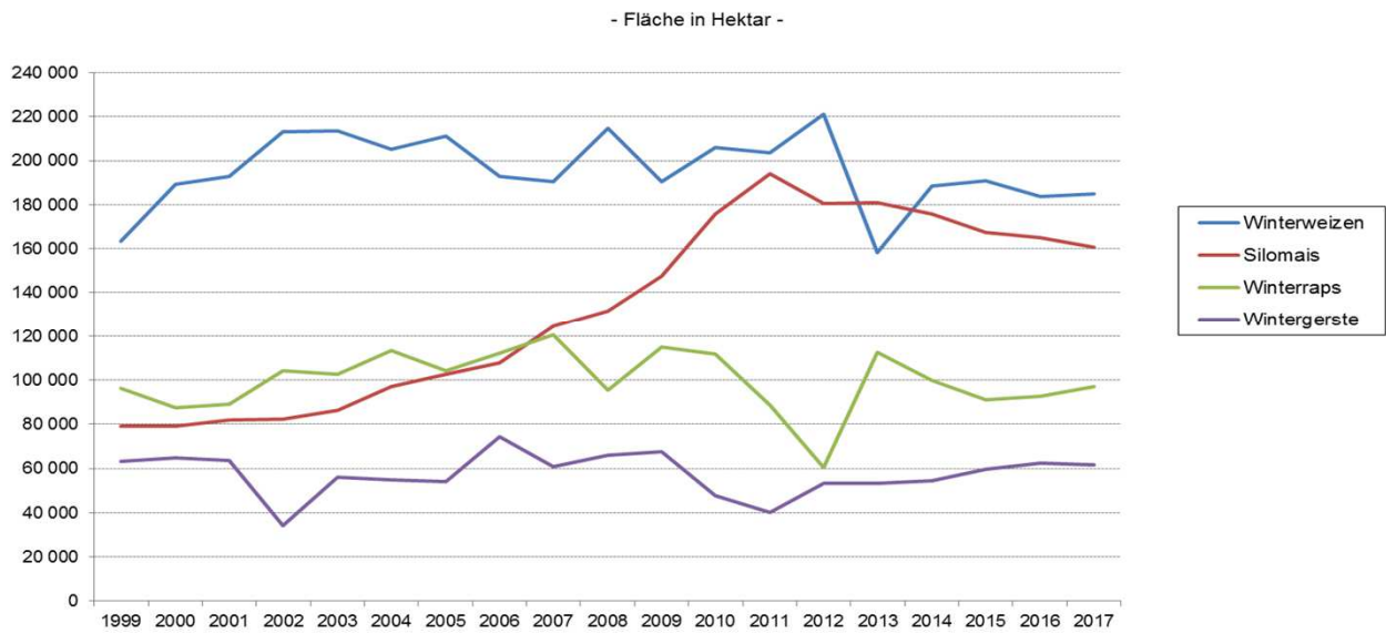
Abb. 1 Entwicklung der Anbaufläche von Winterweizen, Silomais, Winterraps und Wintergerste in Schleswig-Holstein 1999 bis 2017
