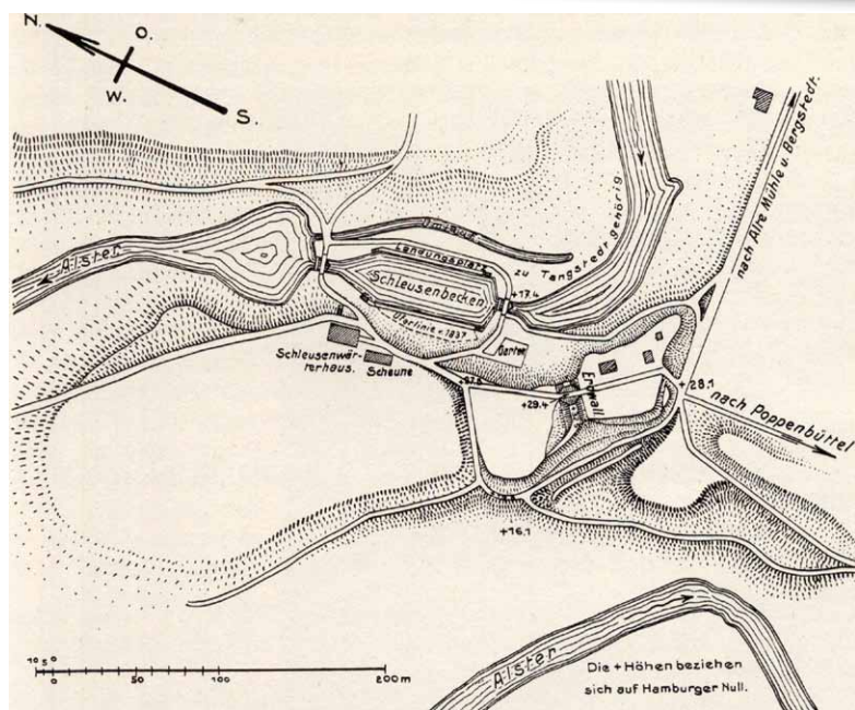
Eine Bauzeichnung mit dem Alsterlauf und genauen Angaben des Schleusenbeckens, des Landungsplatzes und des Schleusenwärterhauses mit Scheune. Heute sind beide Gebäude verbunden.
