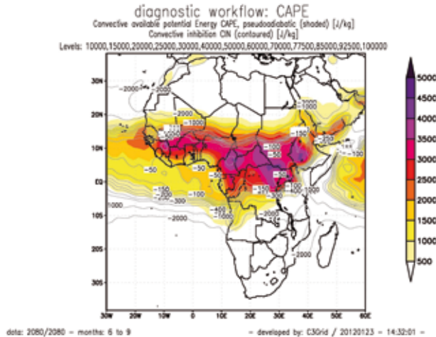
Abb. 3: CAPE: CAPE (Schattierung) und CIN (Konturen) von MPI-ECHAM5/MPI-OM-Simulation mit 1% CO 2 -Anstieg pro Jahr für Juni-September 2080, 1000-100hPa. Hohe CAPE-Werte liegen wie zu erwarten im Bereich der ITCZ, wo hochreichende Konvektion stattfindet. Die hohen CIN-Werte über der Sahara hingegen unterdrücken Konvektion.
