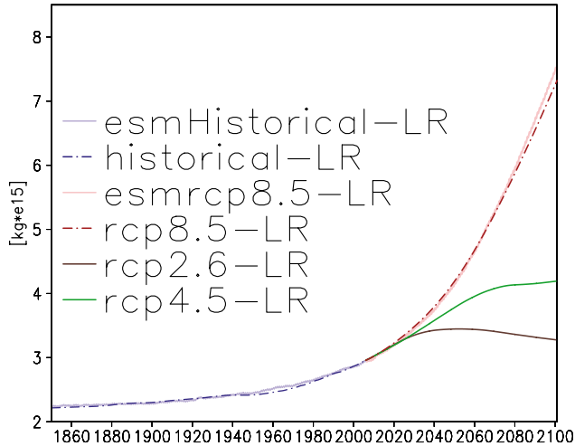
Abb. 5: Zeitliche Entwicklung des Gesamtkohlenstoffs [10 15 kg] in der Atmosphäre, berechnet aus den Werten für das ,historical' und die RCP-Konzentrationsexperimente (grüne, schwarze und gestrichelte Kurven), sowie berechnet mit MPI-ESM-LR in der Projektion des Emissionsszenarios (durchgezogene Kurven in rosa und violett).
