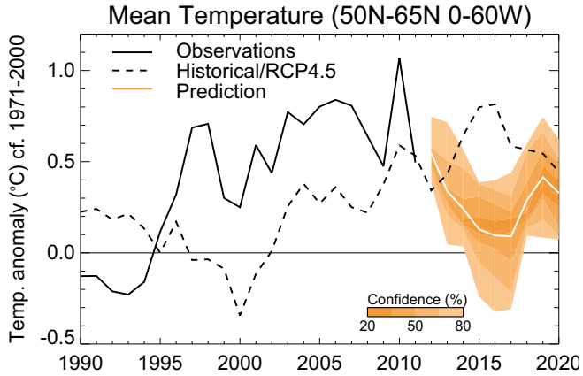
Abb. 4: Jahresmittel der Temperaturanomalien (jeweils Abweichungen vom Mittelwert zwischen 1971 und 2000) an der Ozeanoberfläche im Nordatlantik: Beobachtungen ([3]; durchgezogen, schwarz), Ensemble-Mittel (3 Mitglieder) von ,historical' 1990 bis 2005 und RCP4.5 2006 bis 2020 (gestrichelt, schwarz), Ensemble-Mittel (10 Mitglieder) der dekadischen Vorhersagen 2012 bis 2020 (durchgezogen, weiß). Die verschiedenen Schattierungsgrade um den Mittelwert der dekadischen Vorhersagen zeigen Vertrauensintervalle zwischen 20 und 80 %. (Quelle: Holger Pohlmann, Max-Planck-Institut für Meteorologie)
