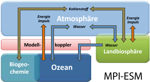
Abb. 1: Schematische Darstellung des Erdsystemmodells MPI-ESM.
