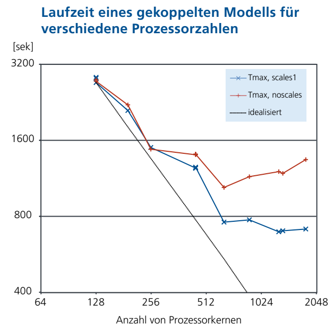
Abb. 1 zeigt ein Beispiel einer niedrig aufgelösten gekoppelten Simulation mit ECHAM/MPI-OM, bei der die Kommunikation bereits mit ScalES-Methoden umgesetzt wurde, so dass der bestmögliche Lauf um 27% beschleunigt wurde (blaue Linie).
