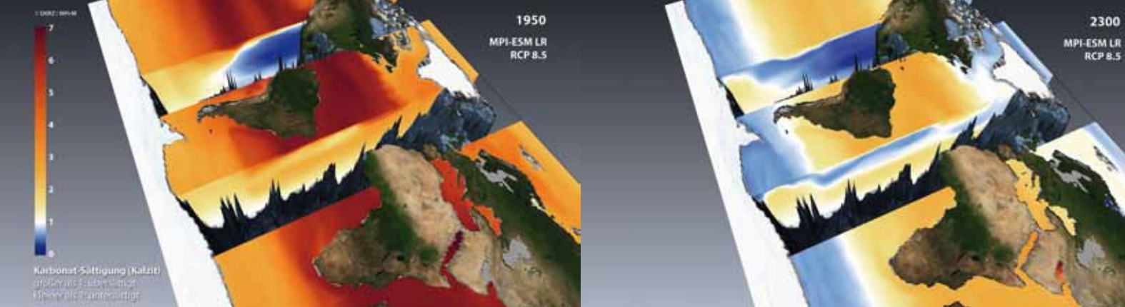
Abb. 6: Karbonatsättigung im Ozean im Jahr 1950 des „historical“ Experiments (links) und im Jahr 2300 des rcp85-Experiments (rechts). Die blau eingefärbten Wassermassen weisen eine Untersättigung auf, die den Abbau von Kalkschalen oder -skeletten bewirken bzw. deren Aufbau behindern würde.
