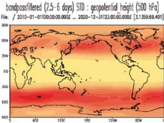
Abb. 2: Das Diagnosewerkzeug stormtrack des C3Grid markiert Regionen mit hoher Sturmaktivität. Diese sind in rot dargestellt.
