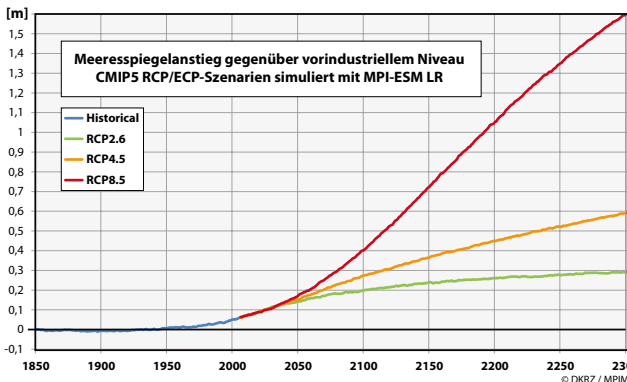
Abb. 3: Simulierter Meeresspiegelanstieg bis 2300 auf Basis der Simulationen mit dem LR-Modell. Ein deutlicher Meeresspiegelanstieg über Jahrhunderte ist zu erwarten: im Jahr 2300 beträgt der mittlere Anstieg je nach Szenario zwischen 0,3 und 1,6 Meter gegenüber dem vorindustriellen Zustand.
