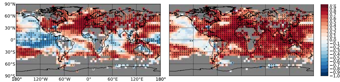
Abb. 1: Um die Qualität des MiKlip-Vorhersagesystems zu beurteilen, werden retrospektive Vorhersagen durchgeführt und mit Beobachtungen verglichen. In der Abbildung wird die Korrelation zwischen der gemittelten Oberflächentemperatur der Vorhersage für die Jahre 2 bis 5 und Beobachtungen gezeigt (blau: keine Vorhersagequalität vorhanden, rot: Vorhersagequalität vorhanden, je dunkler desto besser). Das erste MiKlip System (links) zeigte schlechte Vorhersagequalität in den Tropen, diese konnte im zweiten System (rechts) deutlich verbessert werden.
