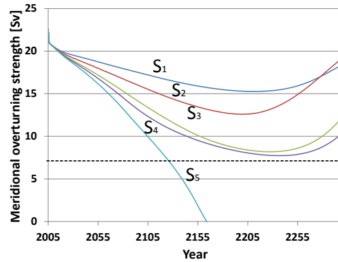
(d) Possible trajectories of the overturning strength
