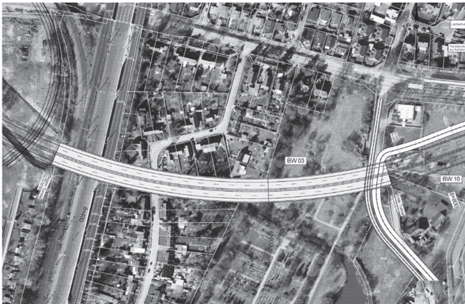
Die A26-Ost käme von Westen unter der Bahn durch, verliefte dann unter dem Katenweg im Tunnel und stiege dahinter zur Otto-Brenner Straße an. Abb.: DEGES/BWVI
