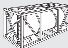
Tank-Container 20' Speziell für flüssige Chemikalien. Ausgewählte Container werden ausschließlich für flüssige Lebensmittel eingesetzt.
