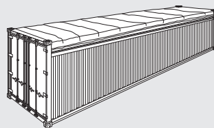
Open Top-Container 20' und 40' Mit abnehmbarer Plane. Speziell für überhohe Ladung. Beladung von oben oder von der Türseite bei ausgeschwenktem Türquerträger.
