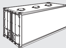
Bulk-Container 20' Speziell für Schüttgut, wie z.B. Malz.
