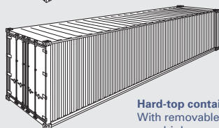
Hardtop-Container 20' und 40' Mit abnehmbarem Stahldach. Speziell für schwere oder überhohe Ladung. Beladung von oben oder von der Türseite bei ausgeschwenktem Türquerträger.
