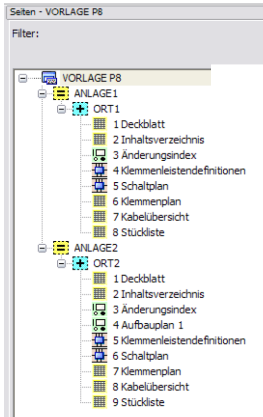
Abbildung 1.: Projektstruktur
