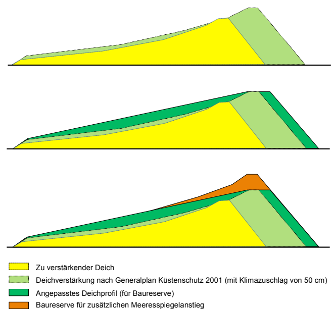
Abb. 7.1.2: Konzept Baureserve für Landesschutzdeiche Schleswig-Holstein-Eintrittswahrscheinlichkeit (HW200) und HW200 + 50 cm (MELUR 2013)
