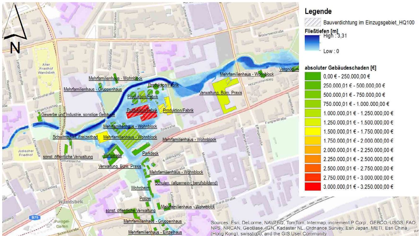
Abb. 5.5.1: Ausschnitt der durch die TUHH durchgeführten Simulation: „Instandsetzungskosten bei einem Hochwasser bei Bauverdichtung des Einzugsgebiets der Wandse in Hamburg“ (D. Friese)
