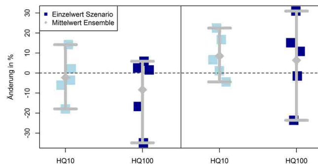
Abb. 7.2.2: Bandbreiten der prozentualen Änderung der Hochwasserabflüsse in der Krückau für verschiedene Wiederkehrintervalle, jeweils dargestellt für 2001 - 2050 (links) und 2051 - 2100 (rechts) gegenüber 1951 - 2000.
