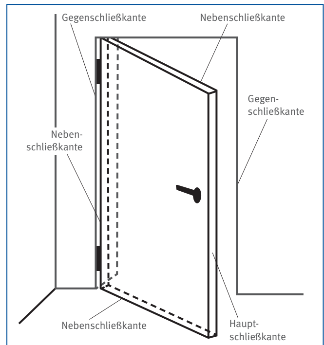
Abbildung 4: Drehflügeltür nach ASR A1.7 (Bundesanstalt für Arbeitsschutz und Arbeitsmedizin – BAuA)
