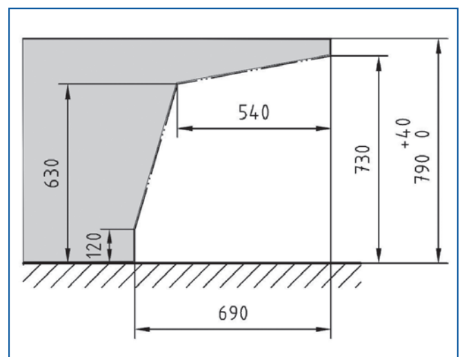
Abbildung 6: Regie- und Produktionsarbeitsplatz (Schnitt)
