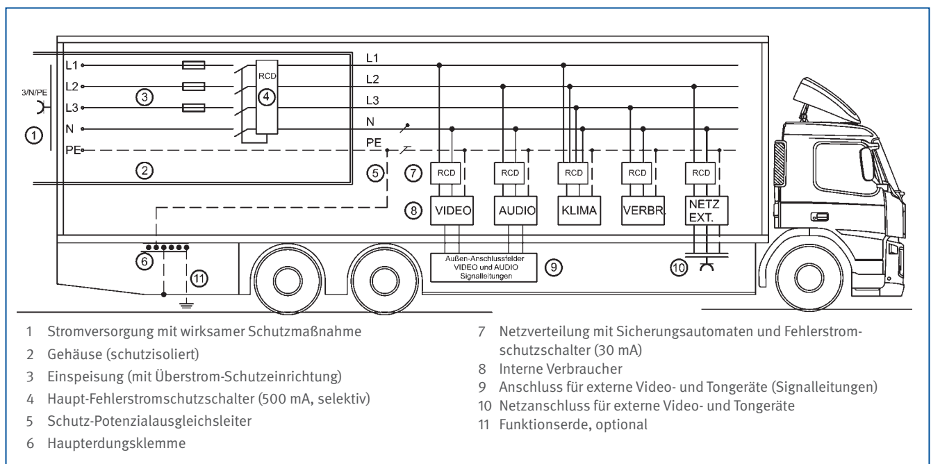
Abbildung 9: Übertragungsfahrzeug ohne Zwischentransformator
