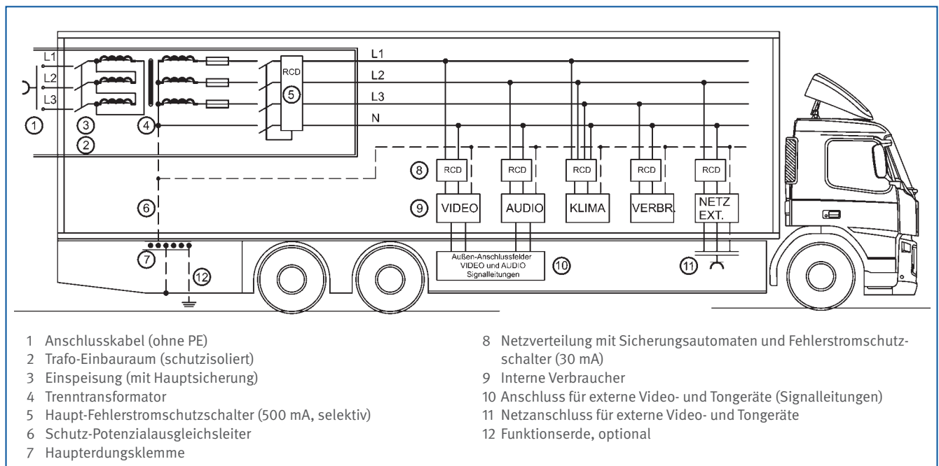
Abbildung 8: Übertragungsfahrzeug mit Zwischentransformator
