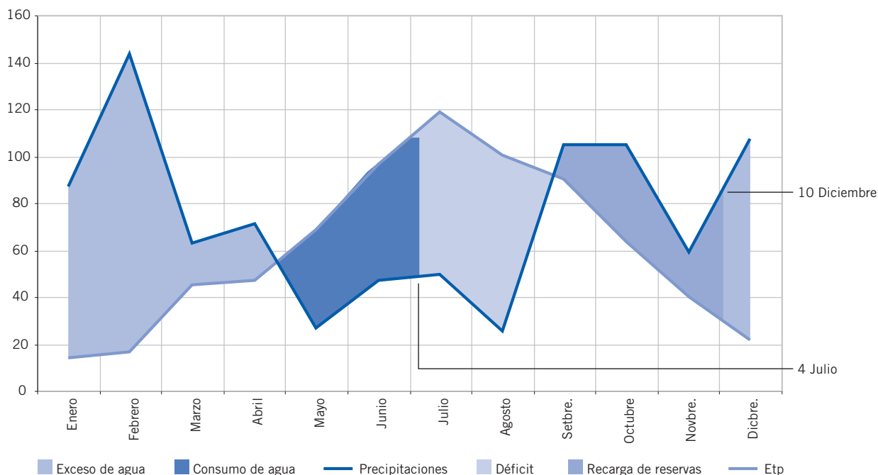
Balance hídrico Año 2006
