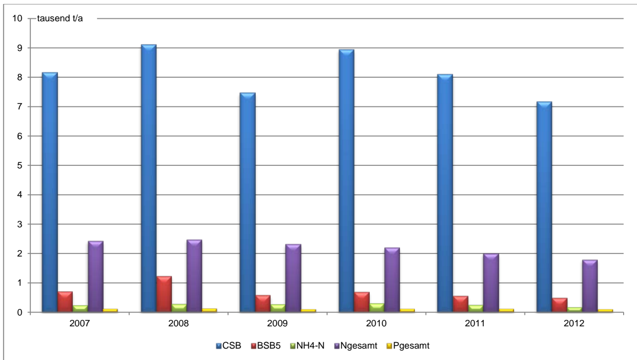
Abbildung 3: Abwasserschmutzfrachten
