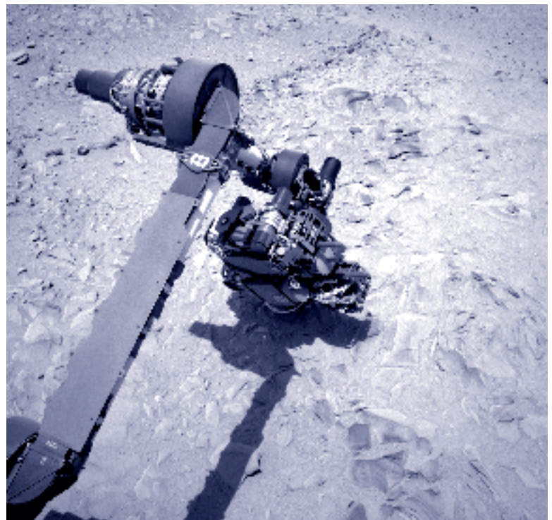
Der Mars Rover Curiosity untersucht den Marsboden
