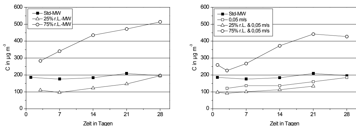
Abbildung 10: Aldehydmissionen von Splintholz, getestet unter Standardbedingungen sowie verschiedenen relativen Luftfeuchten (links) bzw. verringerter Luftgeschwindigkeit und verschiedenen relativen Luftfeuchten (rechts)
