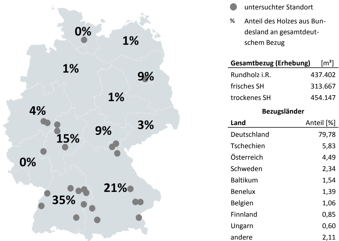
Abbildung 3.2.5.B: Rohholzherkunft für die Herstellung von Konstruktionsvollholz
