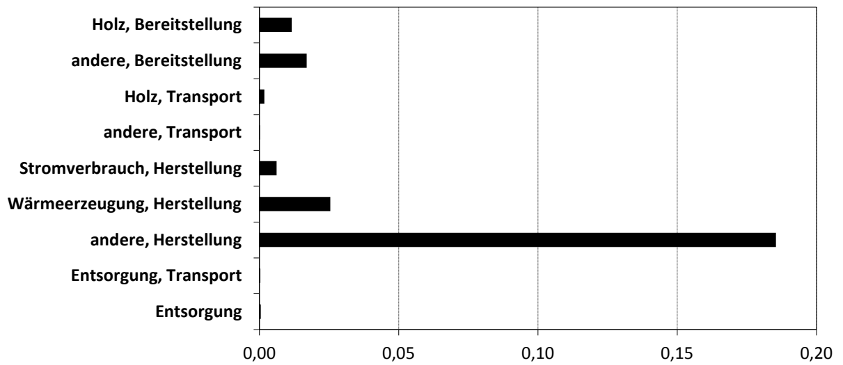
Abbildung 3.2.12.J: Ozonbildungspotential nach Modulen A1 bis A3, C2 und C3 (energetisch) [kg Ethen-Äqv./m 3 Produkt]
