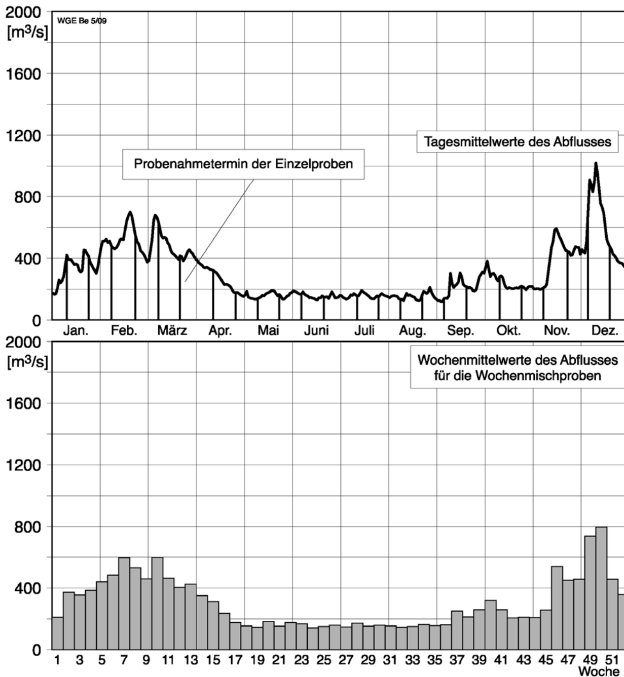
Abfluss der Elbe am Bezugspegel Torgau und die Probenahmetermine 2007 an der Messstelle Dommitzsch
