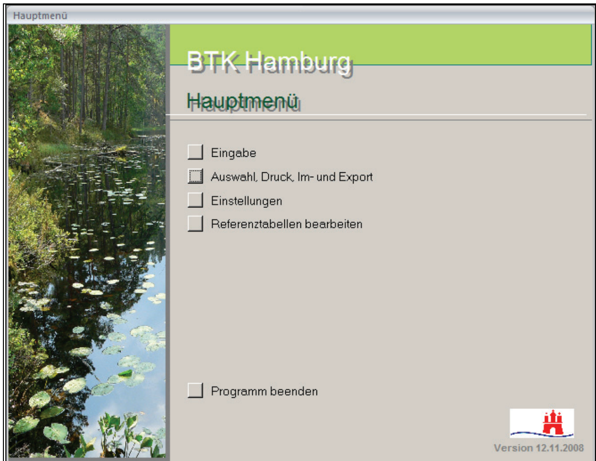
Abb.3 Hauptmenü
