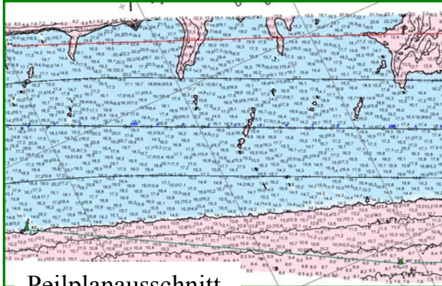
Peilplanausschnitt
