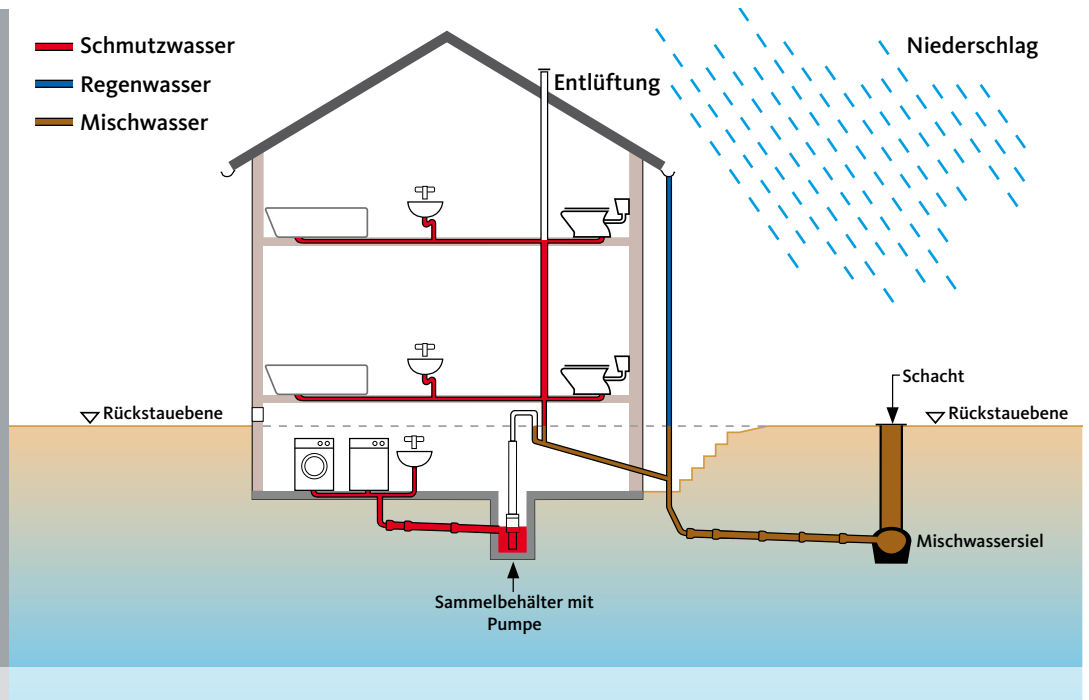
Abbildung 20: Abwasserhebeanlage
